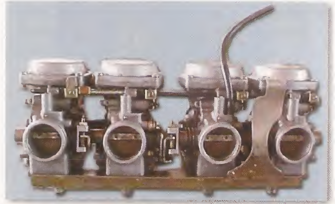
Vista anterior de la batería de carburador de venturi variable
